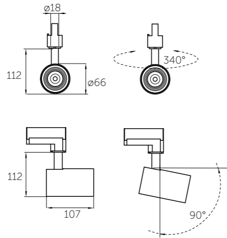
TRACK CON CÁNOPE
