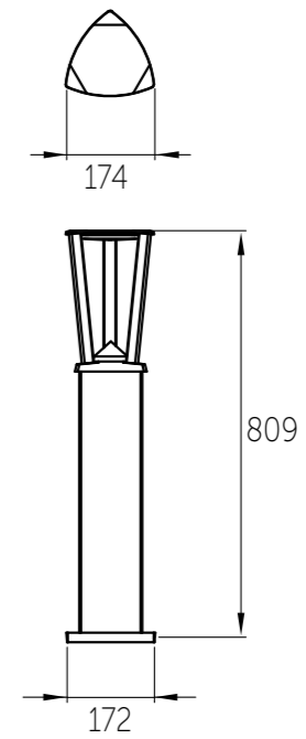
BOLARDO CON DISEÑO EXCLUSIVO CON DIFUSOR FROSTED
