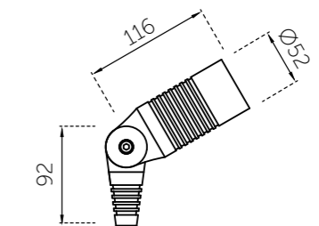
ACABADO EN POLIÉSTER MICROPULVERIZADO TRES LEDS DE ALTA POTENCIA CON SNOOT AJUSTABLE
